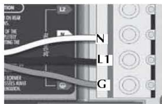
For 120 V (*3 wires)
